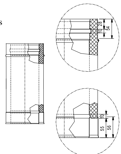
Bild 3: Längenelement
