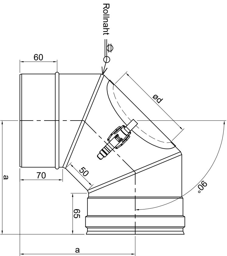
KD mit Viton Dichtung 70ZKT0107
